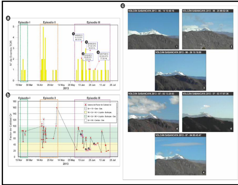
Figura 4.4. Correlación entre: a. Ocurrencia de los eventos Tornillo, b. Valores estimados para el factor de calidad Q_r y f. c. Actividad superficial. Volcán Sabancaya, durante marzo – julio del 2013.
