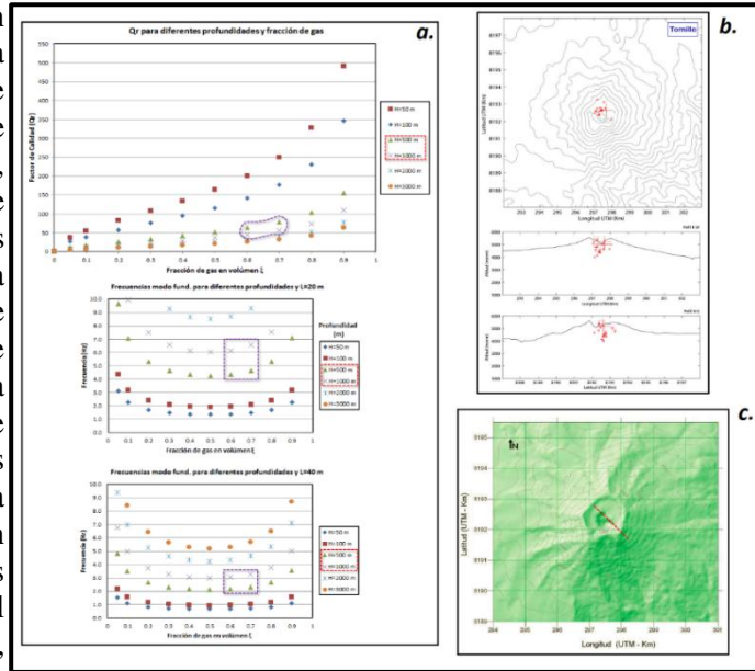
Figura 4.2. Modelamiento de Q_r y f para diferentes profundidades y fracciones de volumen de gas (Roberto Torres et al., 1977, 1978); b. Distribución espacial de los sismos Tornillos, volcán Ubinas, marzo – abril del 1998 (Taipe, 2008); c. Falla del volcán Ubinas (Rivera, 1997) y la posible fuente generadora de los Tornillo (Taipe, 2008).
