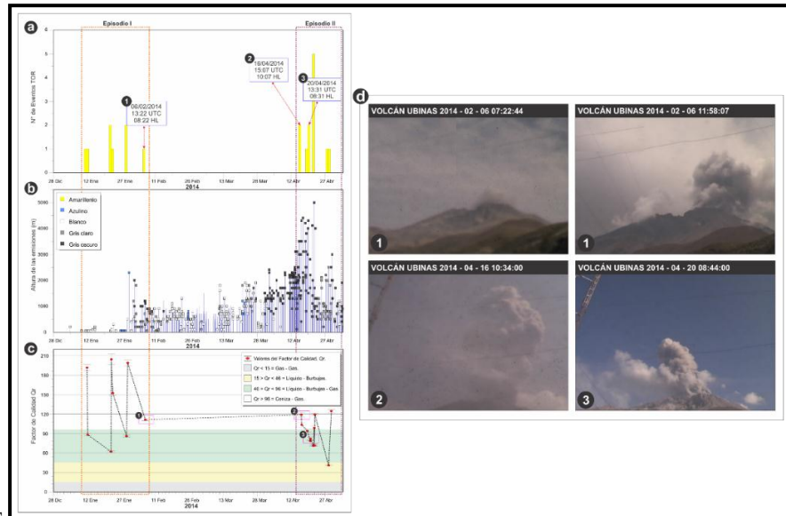
Figura 4.5. Correlación entre: a. Ocurrencia de los eventos Tornillo, b. Altura y coloración de las emisiones, c. Valores estimados para el factor de calidad Q_r y f , d. Actividad superficial. Volcán Ubinas, durante enero –
