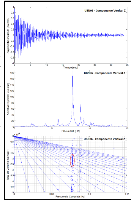
Figura 3.1. Análisis SOMPI a la señal de tipo Tornillo registrada el día 29/01/2014 por la estación UBN06 (volcán Ubinas) componente vertical (Z).
