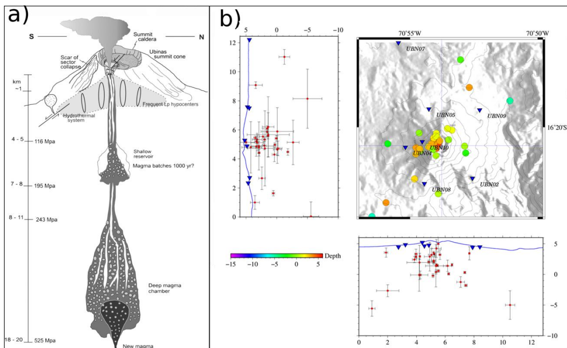
Figura 4. a) Sección transversal esquemática que ilustra el sistema magmático del volcán Ubinas (Rivera et al. 2014). b) Mapa de localización de sismos tipo VT de fase presurización, y sus respectivos perfiles en profundidad (los triángulos azules representan la ubicación de las estaciones sísmicas, y los círculos la fuente sísmica).
