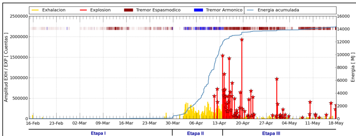
Figura 3. Evolución de la actividad sísmica del volcán Ubinas, correspondiente al proceso eruptivo del 2014.
