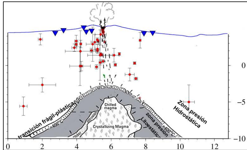
Figura 5. Modelo esquemático del sistema magmático del volcán Ubinas, interpretados a partir de datos sísmicos y estudios petrológicos (en círculo rojo se representa los sismos tipo VT).
