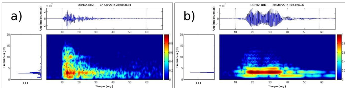
Figura 2. Características sísmicas (forma de onda, espectro y espectrograma) de señales precursoras de ascenso de magma registradas en la estación UBN02. a) Evento sísmico tipo Híbrido, b) evento sísmico tipo Tremor Armónico. El color decodificación dado, representa la densidad espectral de la amplitud normalizada de la onda sísmica
