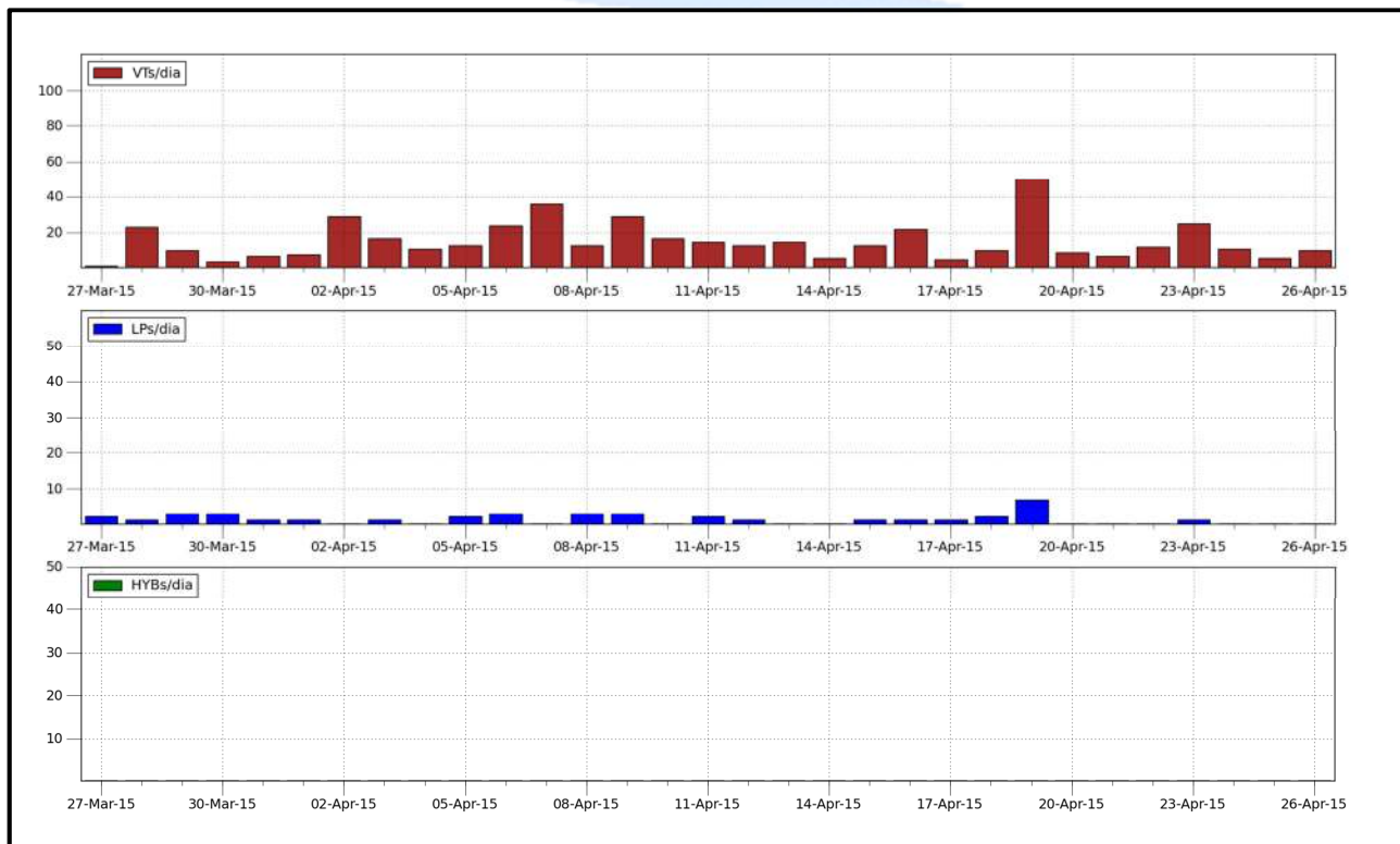
Figura 1.1. Cuadro estadístico de la actividad sísmica del volcán Misti, registrado entre los días 27/03/2015 y 26/04/2015. VT: sismo volcano-tectónico, asociado al fracturamiento de rocas. LP: sismo de largo periodo, asociado a la circulación de fluidos. HYB: sismo híbrido, asociado al ascenso de magma.
