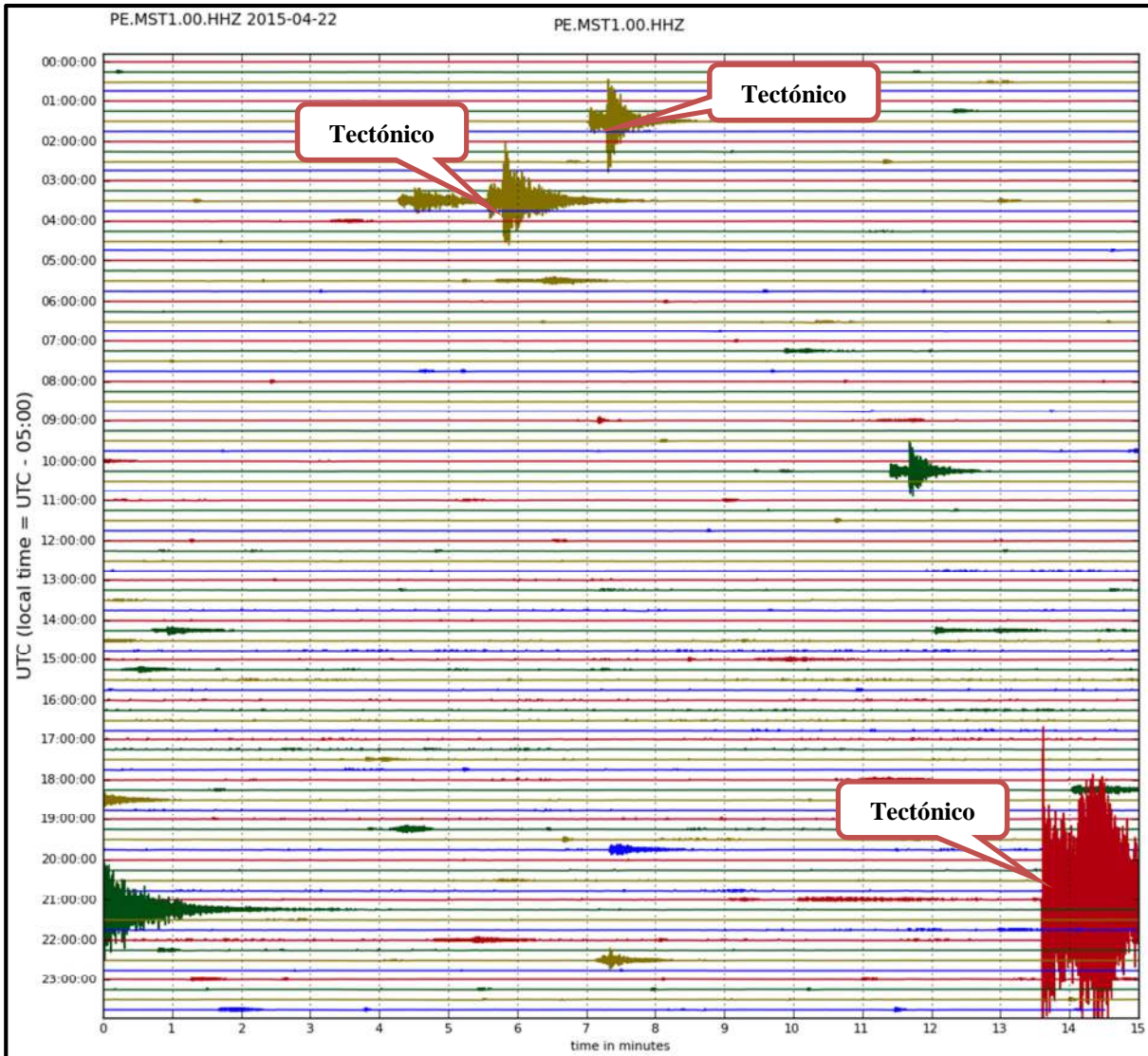
Figura 1.2. Actividad sísmica del volcán Misti correspondiente al día 22 de abril del 2015 (tiempo UTC).
