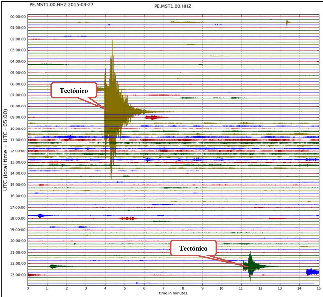
Figura 1.2. Actividad sísmica del volcán Misti correspondiente al día 27 de abril del 2015 (tiempo UTC).
