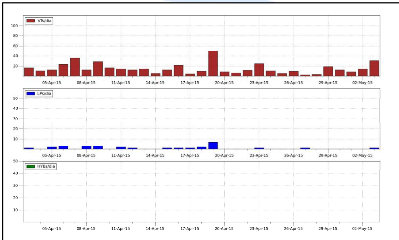
Figura 1.1. Cuadro estadístico de la actividad sísmica del volcán Misti, registrado entre los días 03/04/2015 y 03/05/2015. VT: sismo volcano-tectónico, asociado al fracturamiento de rocas. LP: sismo de largo periodo, asociado a la circulación de fluidos. HYB: sismo híbrido, asociado al ascenso de magma.
