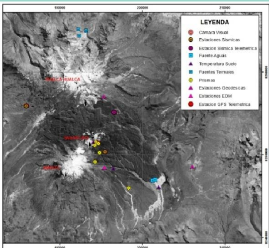
Red de monitoreo del volcán Sabancaya
