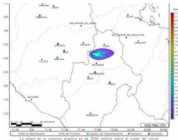
Mapa de pronóstico de dispersión de ceniza.
