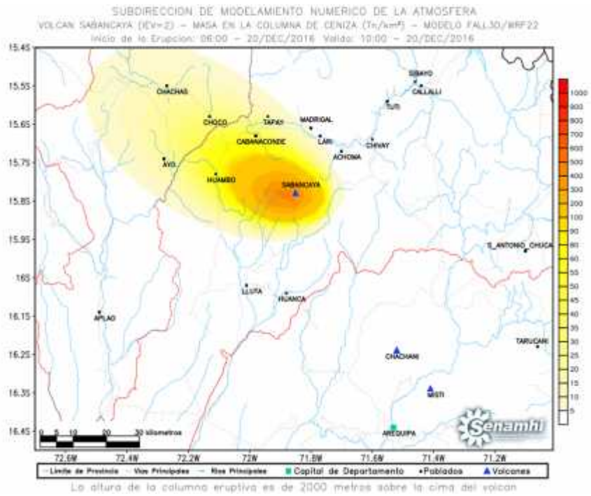
Imagen de la dirección de la dispersión de ceniza
